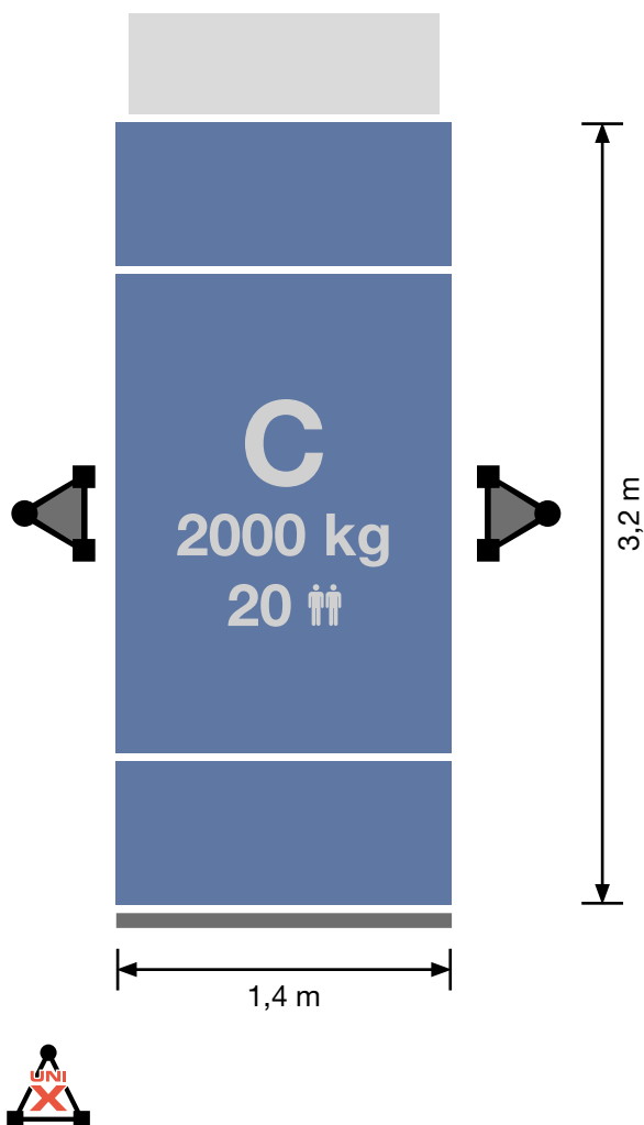
GEDA MULTILIFT P18 Bühne C 1 Beladeschiebetür / 1 Entladerampe
